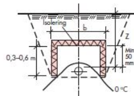
Figur 23. Hästskoformad isolering.
